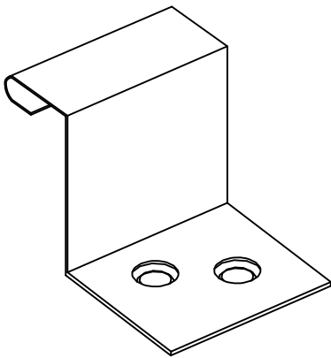
NedZink® Standing Seam Fixed Clip
