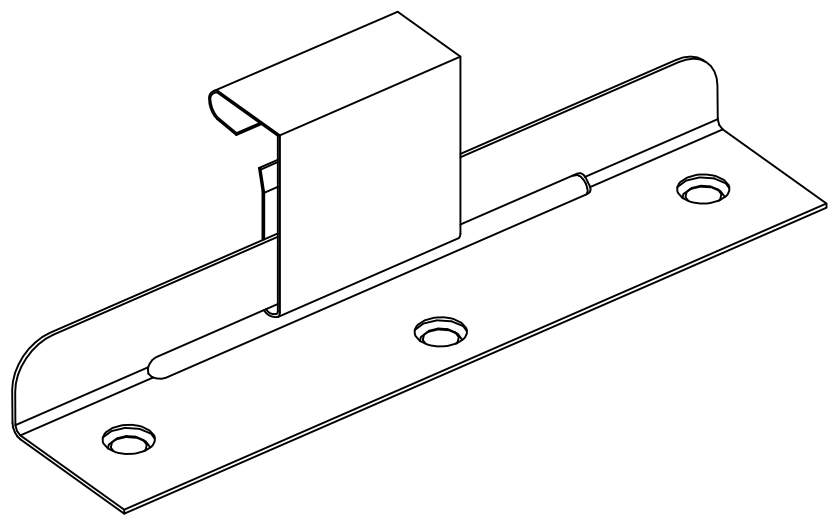
NedZink® Standing Seam Sliding Clip
